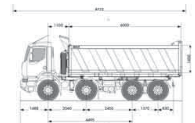
Renault Kerax 8 x 4
