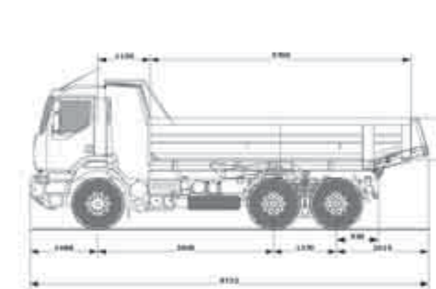
Renault Kerax 6 x 4
